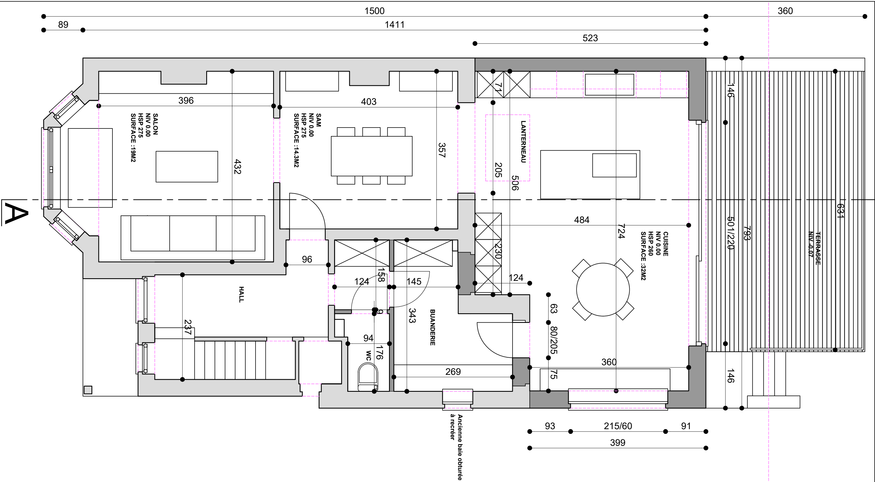
SITUATION PROJETE échelle: 1/ 50 PLAN DU REZ DE CHAUSSEE
