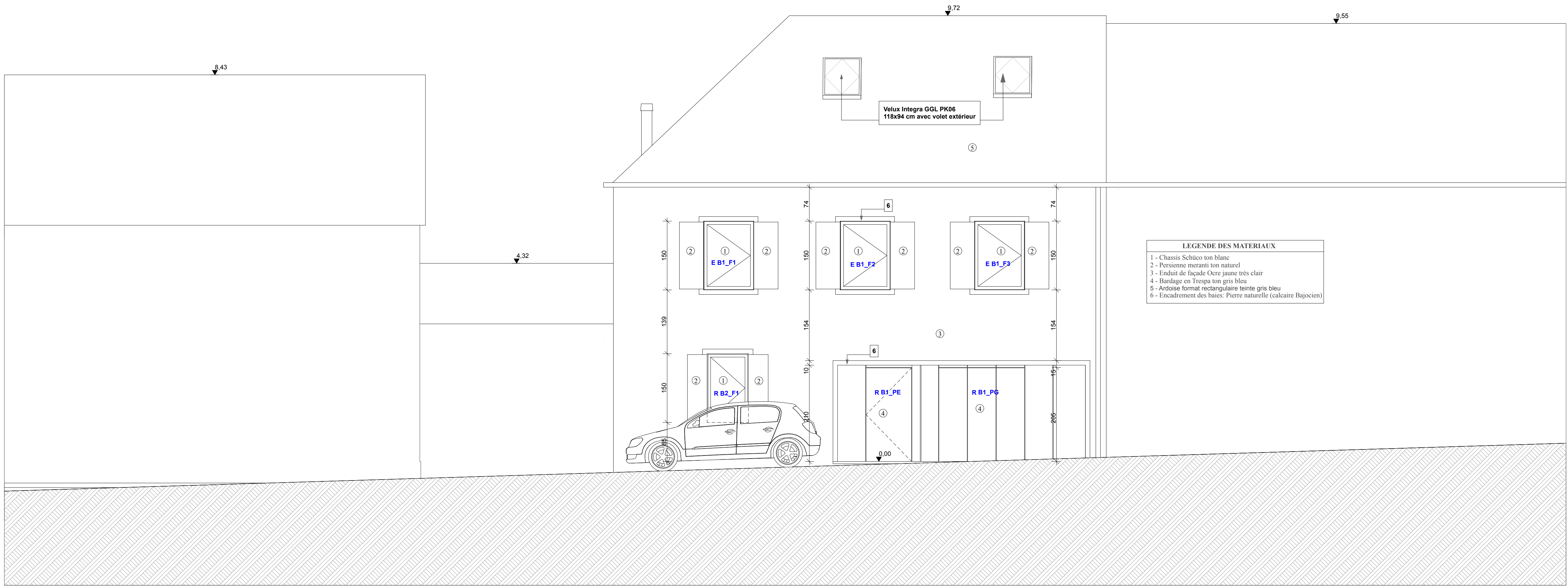
FACADE AVANT
