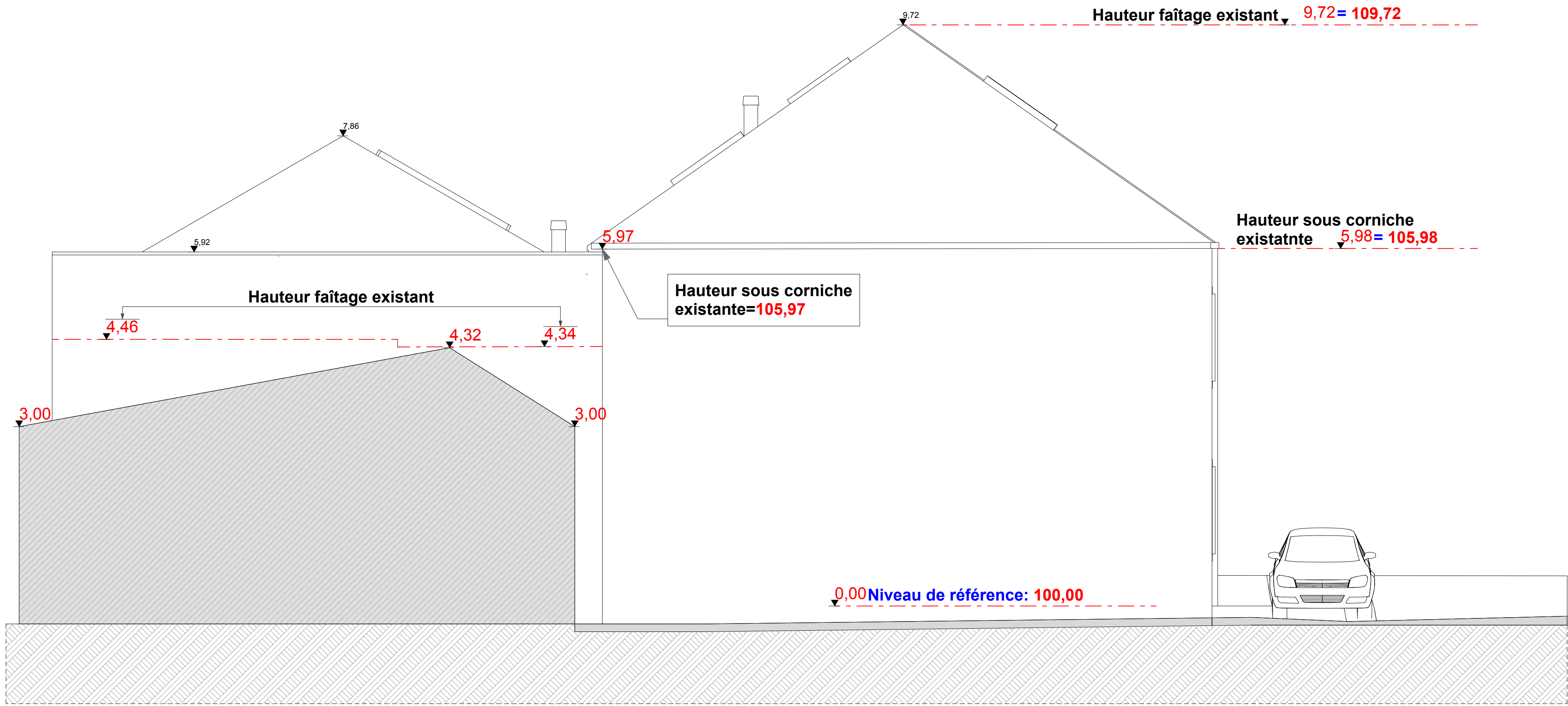
FACADE LATTERALE GAUCHE
