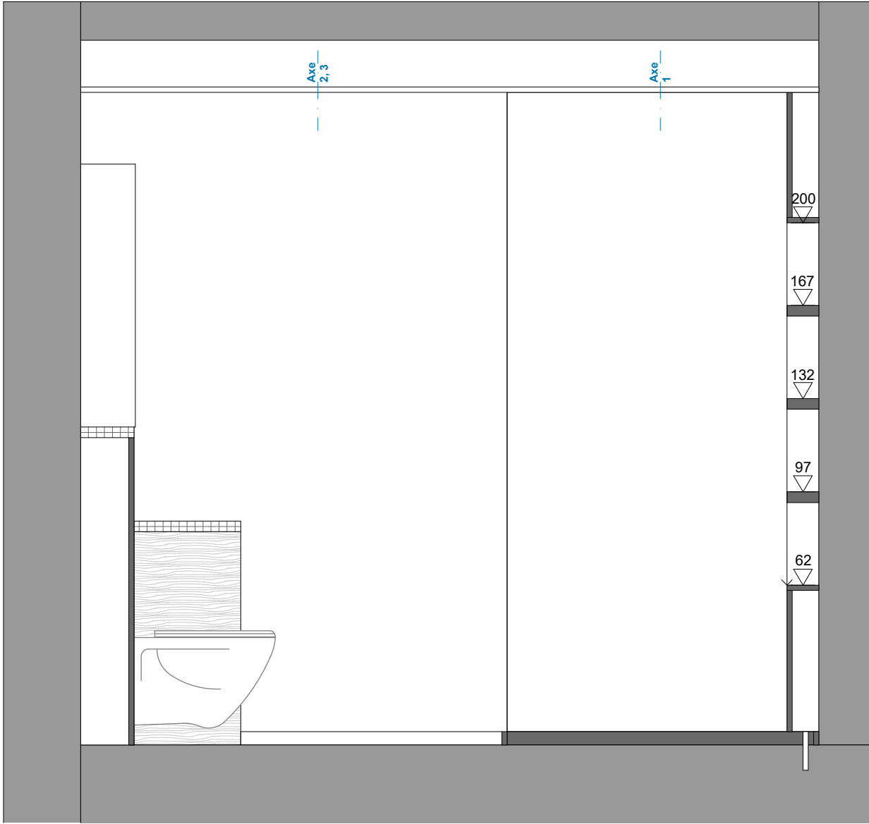
COUPE CC
