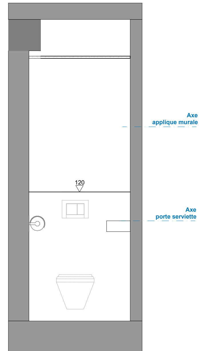
COUPE BB
