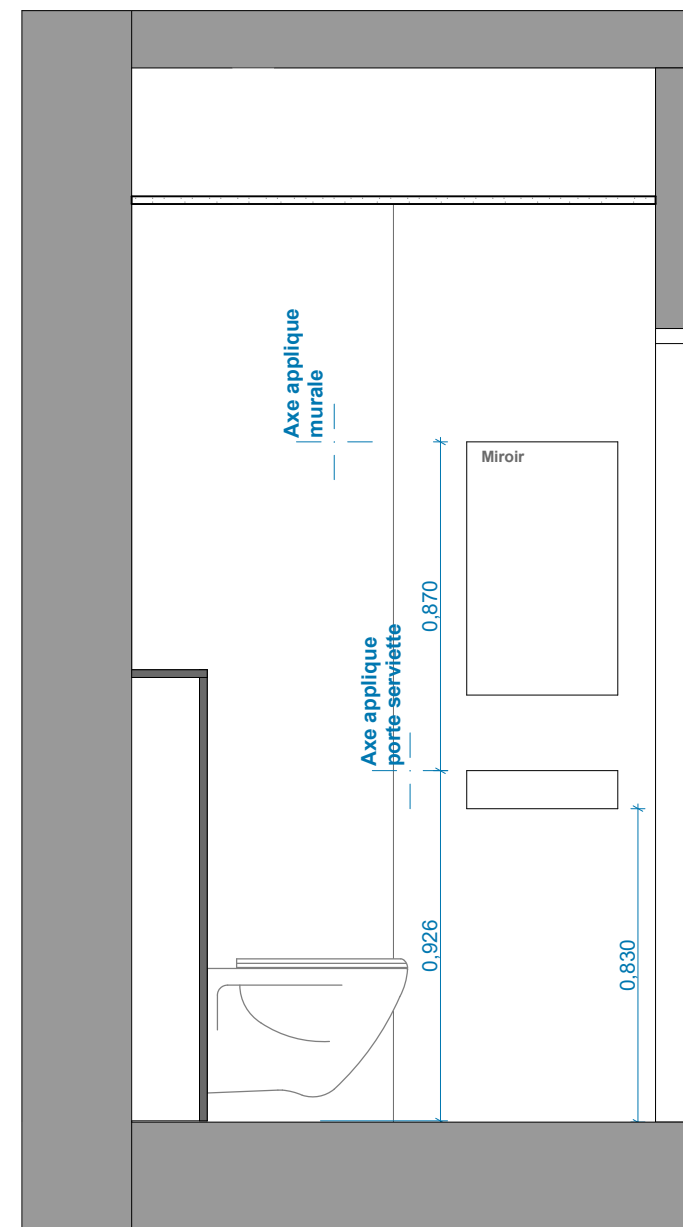
COUPE AA
