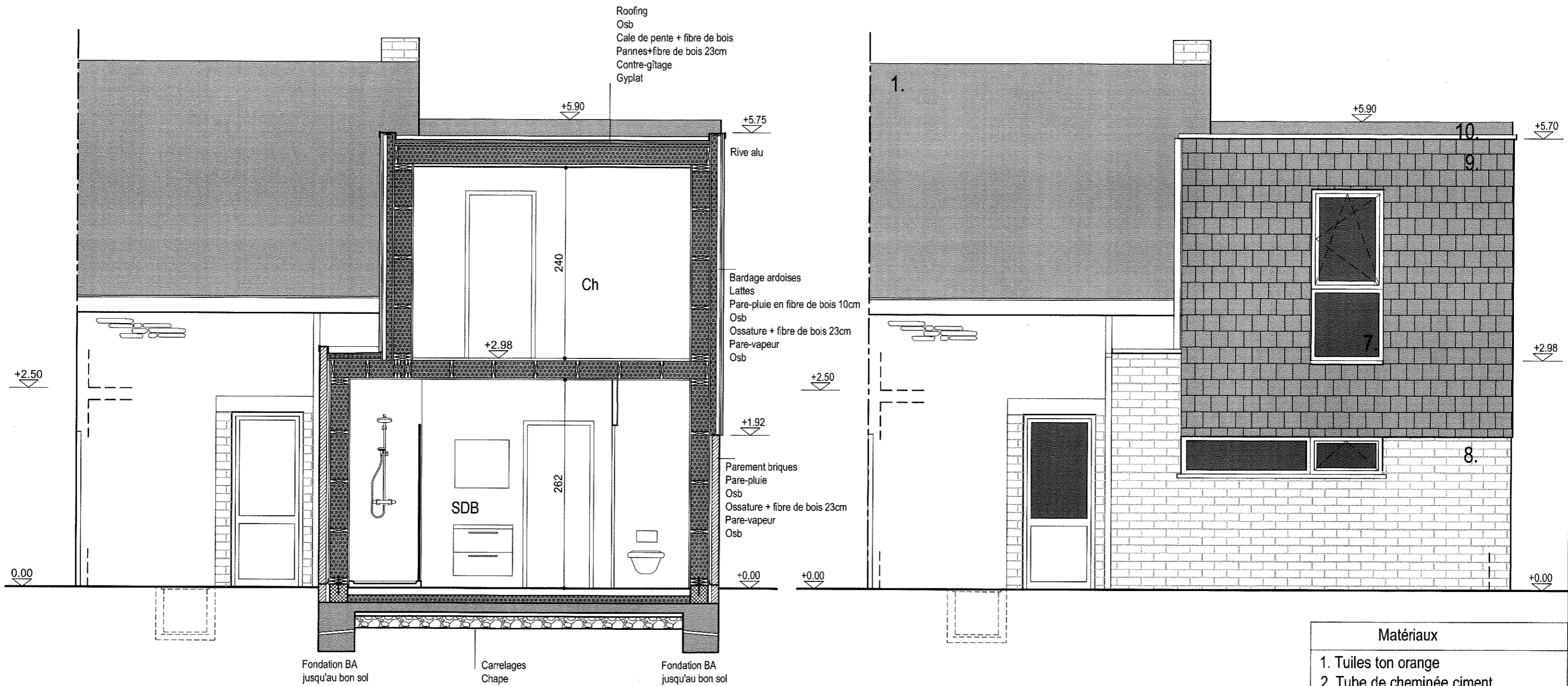
Coupe BB projetée - 1/50
