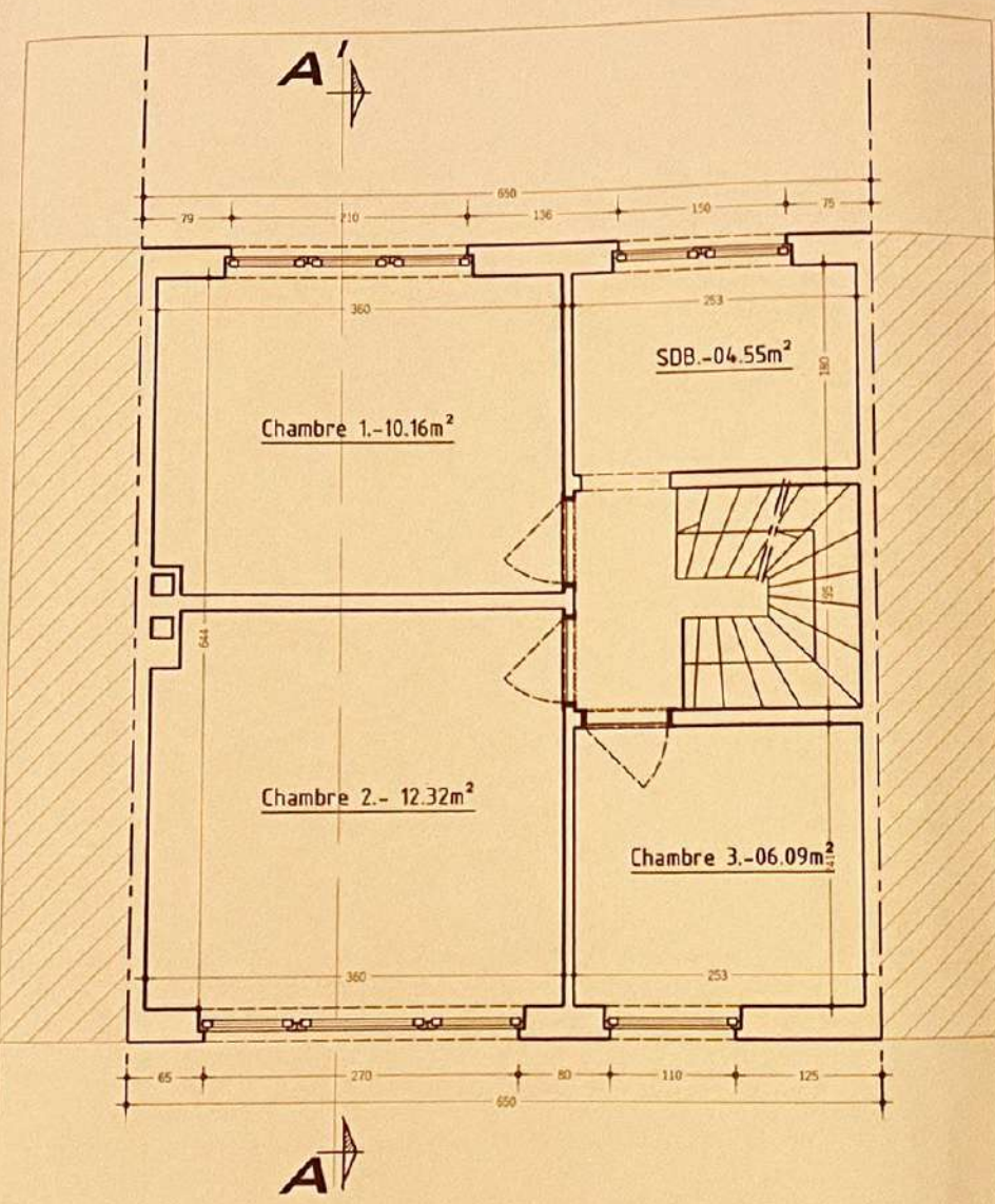
Plan : REZ+2 Ech 1/50
