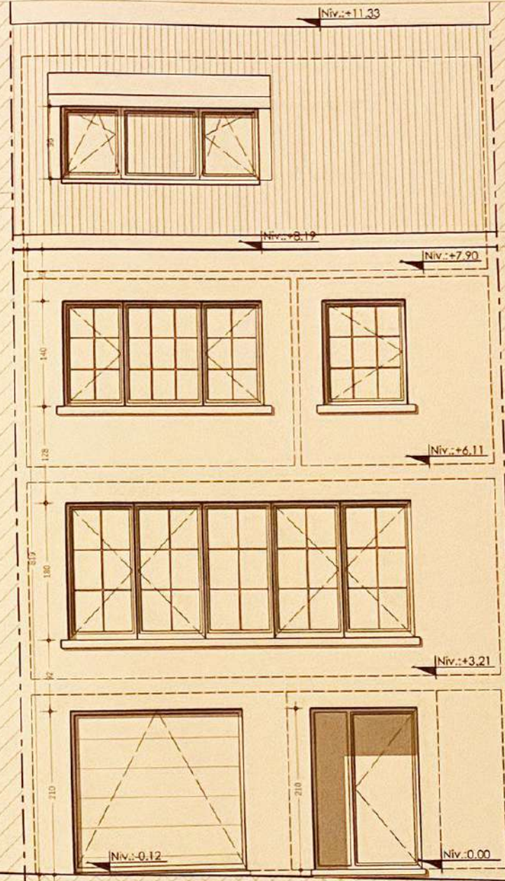
Façade arrière Ech 1/50
