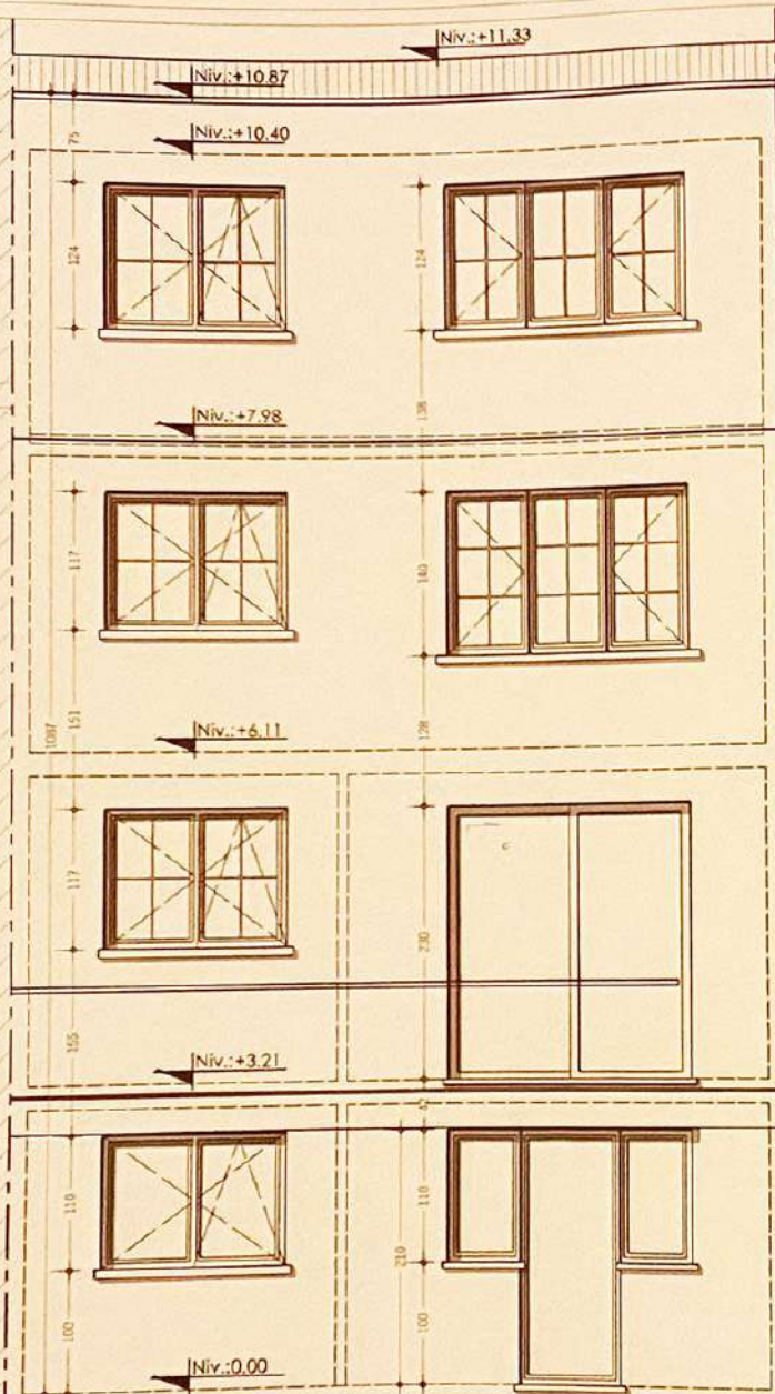
Façade avant Ech 1/50
