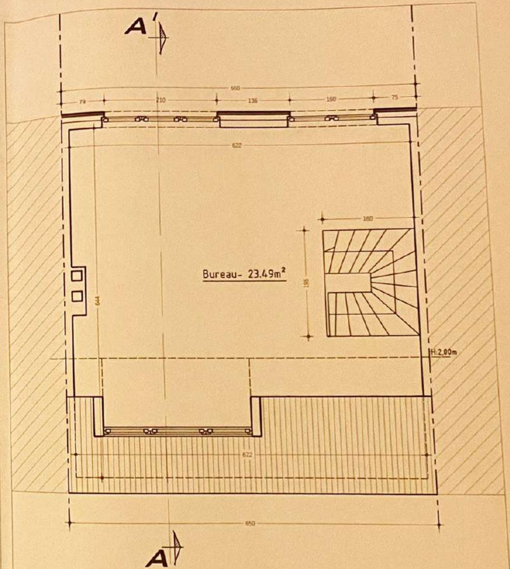
Plan : Combles Ech 1/50
