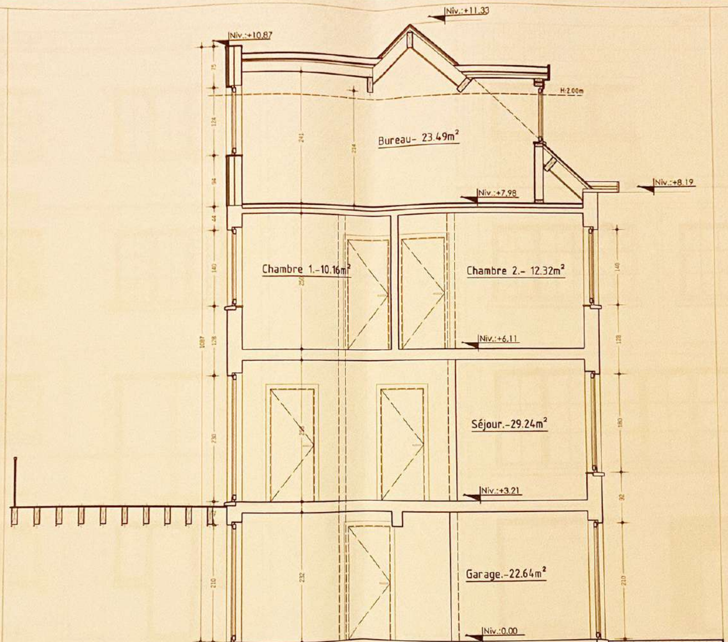
Coupe AA' Ech 1/50
