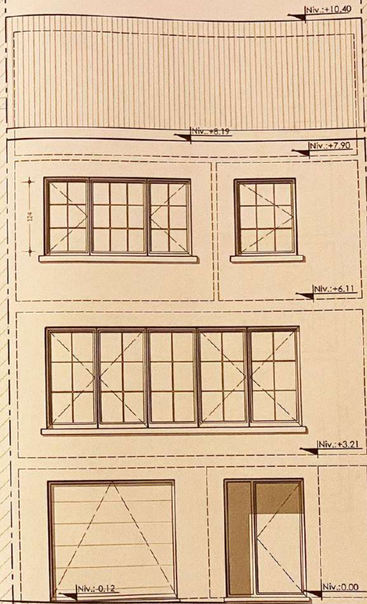
Façade arrière Ech 1/50
